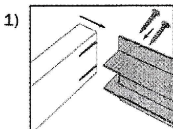
Overstykket samles med bagstykket. Brug 2 stk. 4,5x25 mm skruer.
