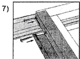
Fastgør derefter støtteskinerne til topstykket med 4,5x25 mm skruer.
