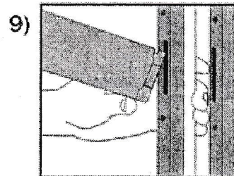
Til gips skal metalsiden af tværstiverne vende udad (brug 19 mm gipspladeskruer). Fastgør først tværstiverne i støtteskinen.
