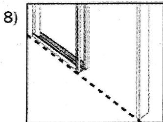
Ret gulvprofilen ind. Støttelisterne skal være i lod. Fastgør gulvprofilen til gulvet med 4 stk. 4,5x25 mm skruer.
