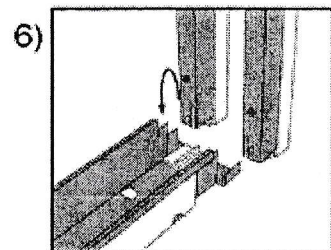
Støtteskinerne skal placeres ind i gulvprofilen som vist.
